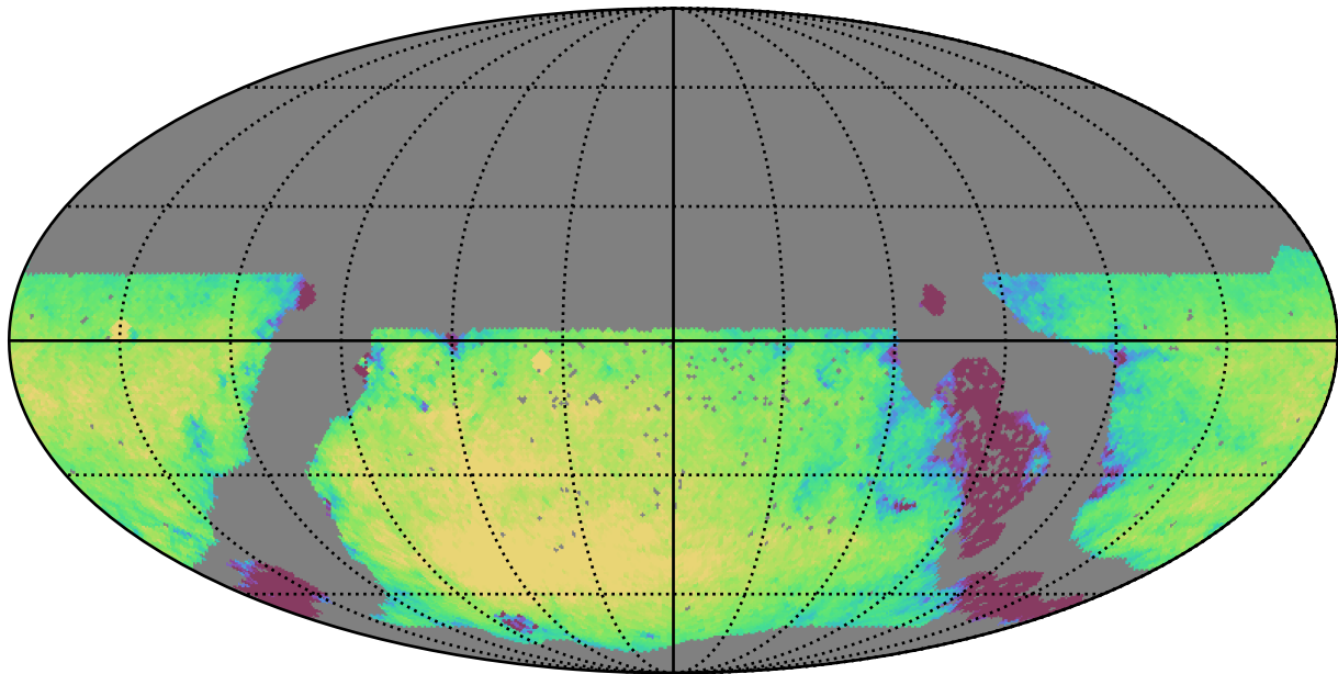
no_long_daily_v3.4_10yrs WFD g band: Exgal_CoaddM5
