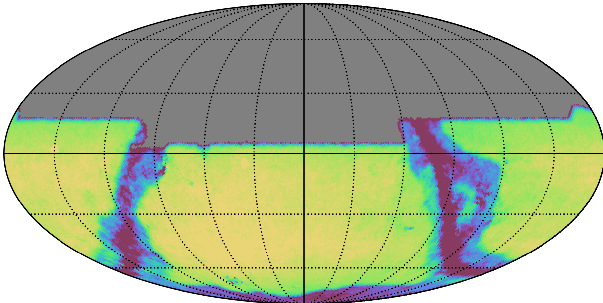
no_long_daily_v3.4_10yrs All sky y band: Exgal_CoaddM5
