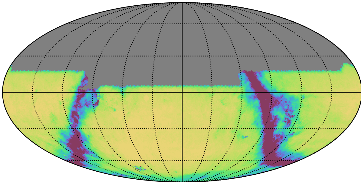
no_long_daily_v3.4_10yrs All sky u band: Exgal_CoaddM5
