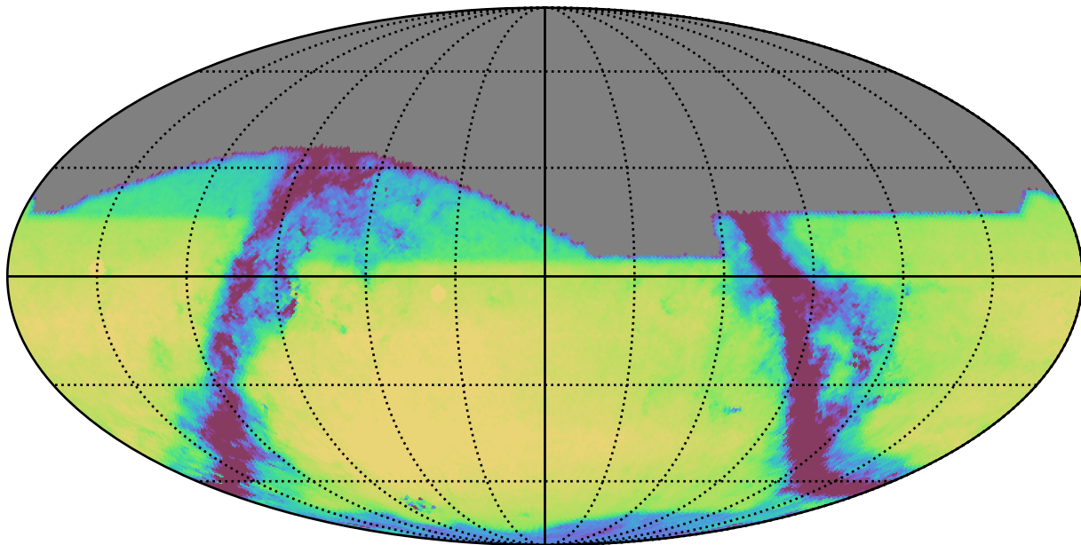
no_long_daily_v3.4_10yrs All sky r band: Exgal_CoaddM5
