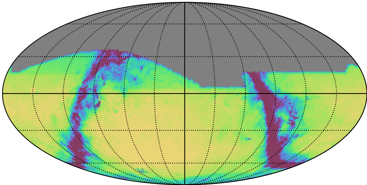
no_long_daily_v3.4_10yrs All sky g band: Exgal_CoaddM5
