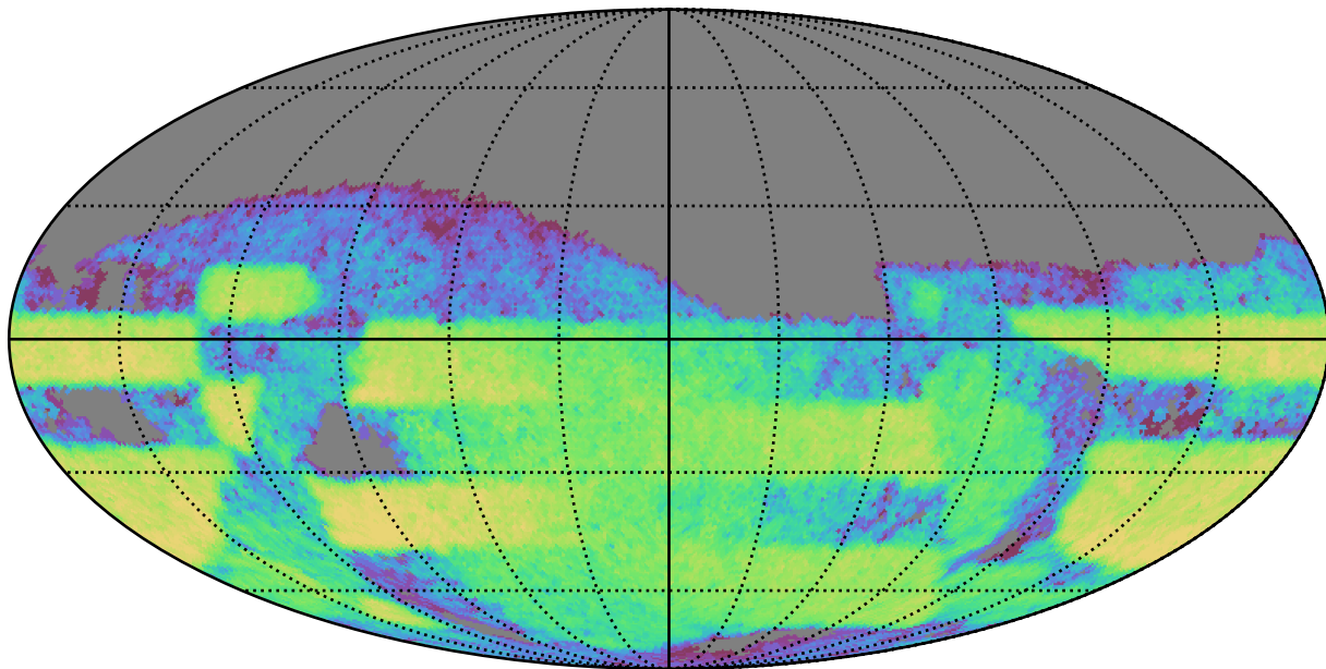
no_long_daily_v3.4_10yrs Yr 3-4 z band: CoaddM5
