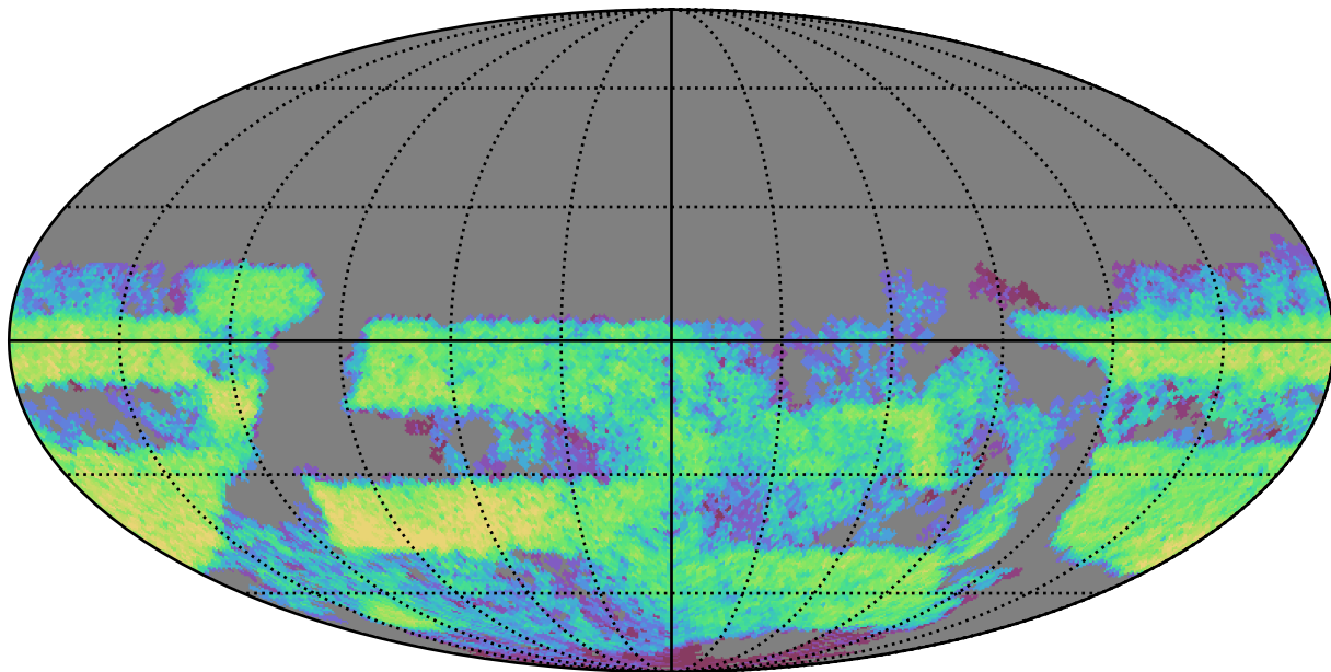
no_long_daily_v3.4_10yrs Yr 3-4 u band: CoaddM5
