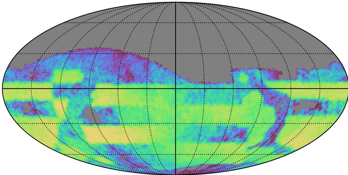
no_long_daily_v3.4_10yrs Yr 3-4 r band: CoaddM5
