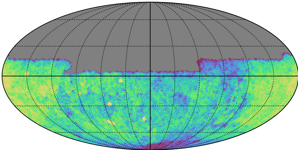
no_long_daily_v3.4_10yrs Yr 1 u band: CoaddM5
