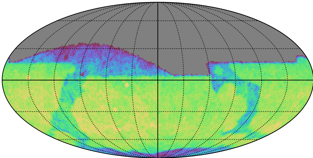
no_long_daily_v3.4_10yrs Yr 1 r band: CoaddM5
