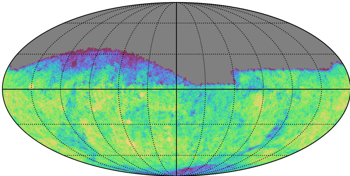
no_long_daily_v3.4_10yrs Yr 1 g band: CoaddM5
