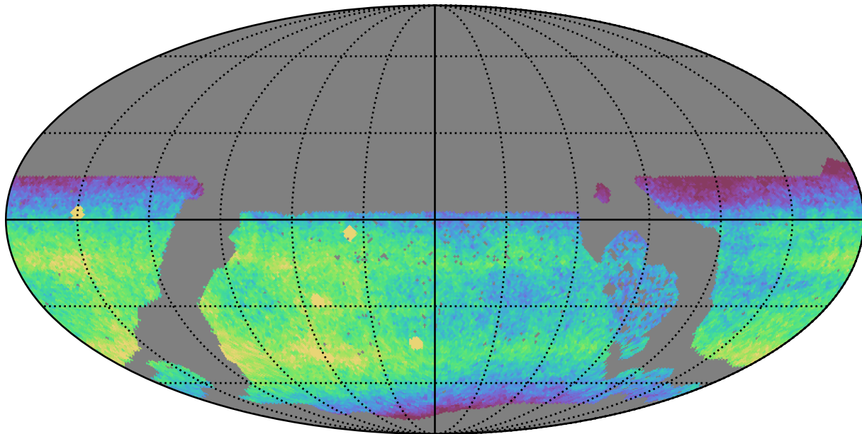
no_long_daily_v3.4_10yrs WFD z band: CoaddM5
