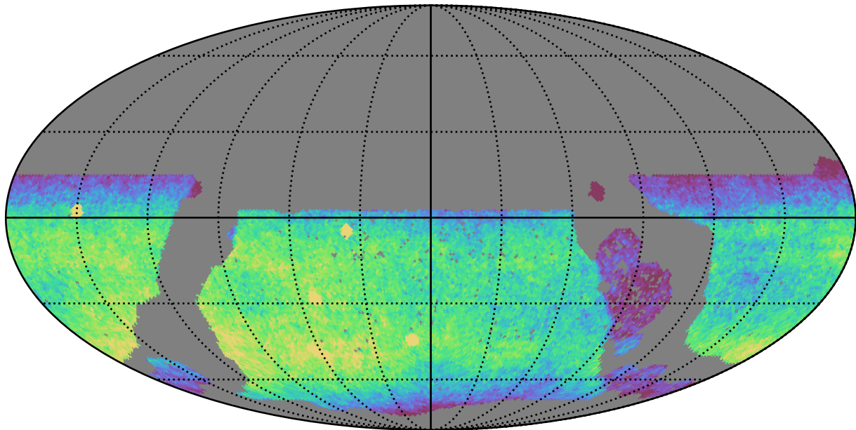
no_long_daily_v3.4_10yrs WFD y band: CoaddM5
