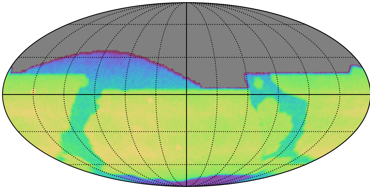
no_long_daily_v3.4_10yrs All sky z band: CoaddM5
