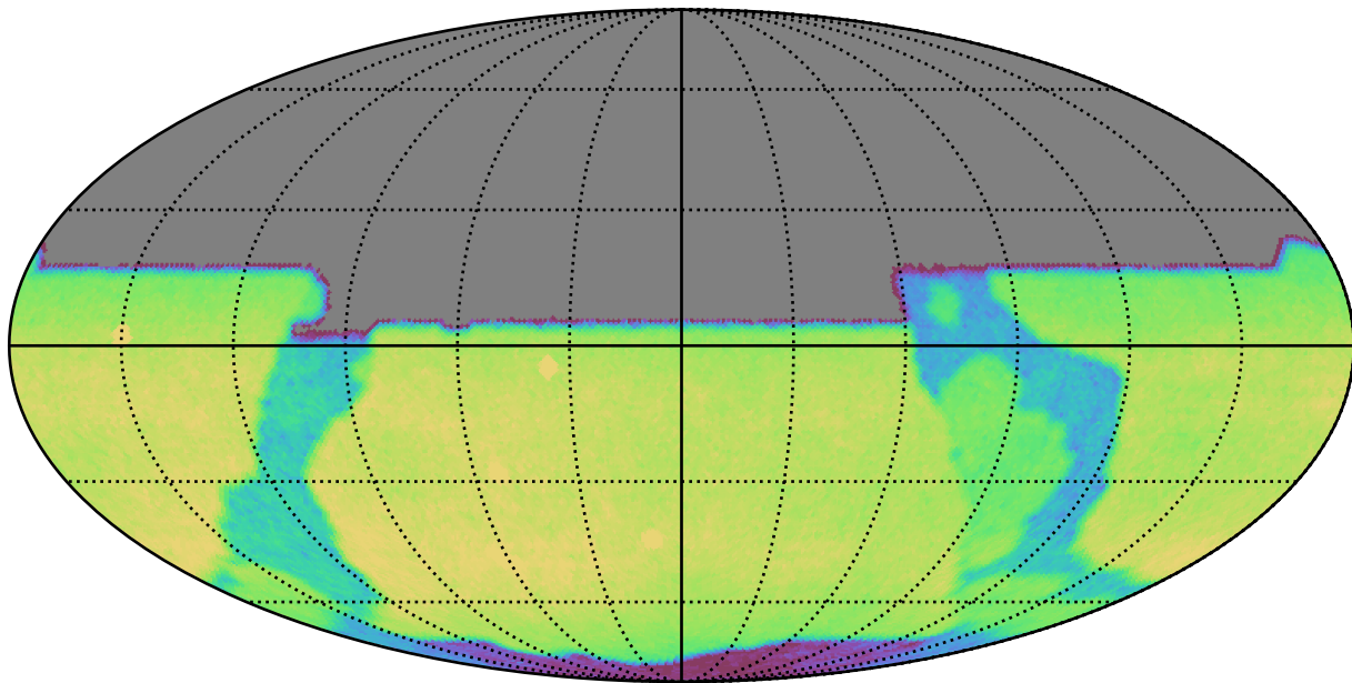
no_long_daily_v3.4_10yrs All sky y band: CoaddM5
