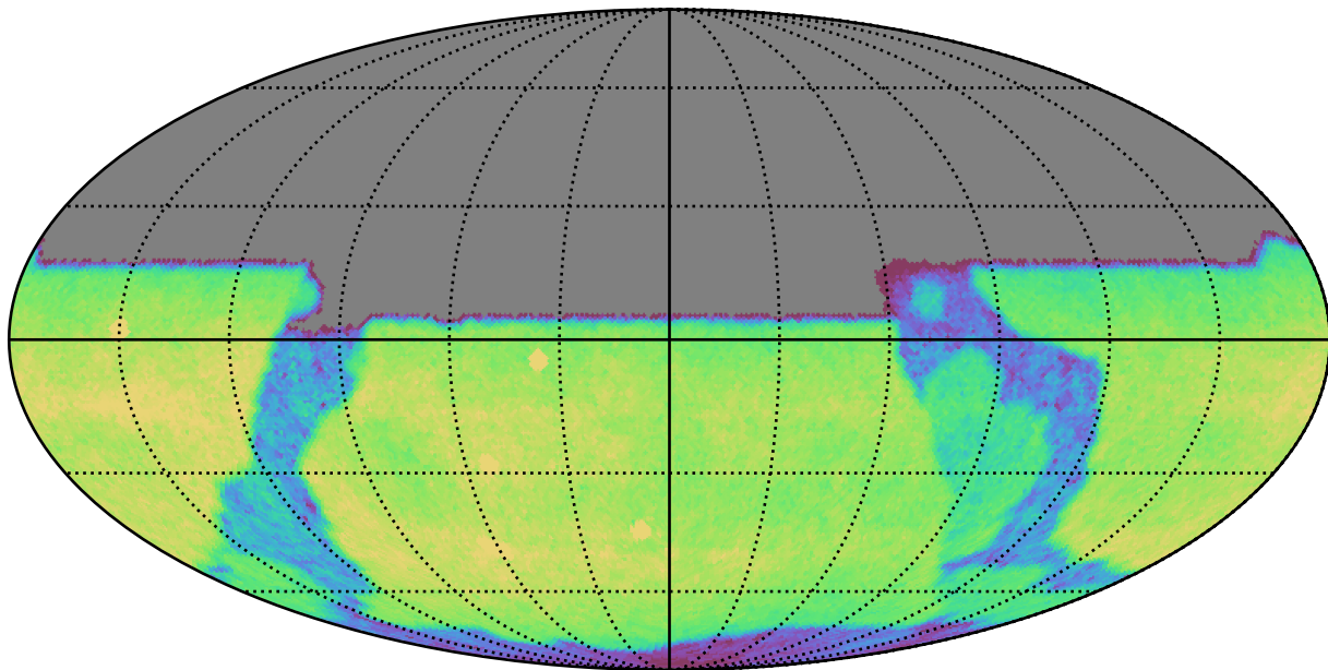
no_long_daily_v3.4_10yrs All sky u band: CoaddM5
