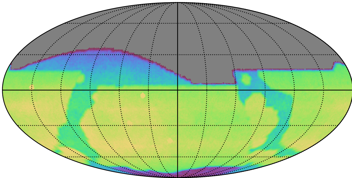
no_long_daily_v3.4_10yrs All sky r band: CoaddM5
