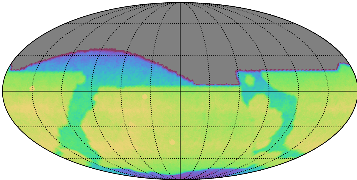
no_long_daily_v3.4_10yrs All sky i band: CoaddM5
