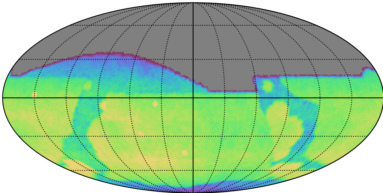
no_long_daily_v3.4_10yrs All sky g band: CoaddM5
