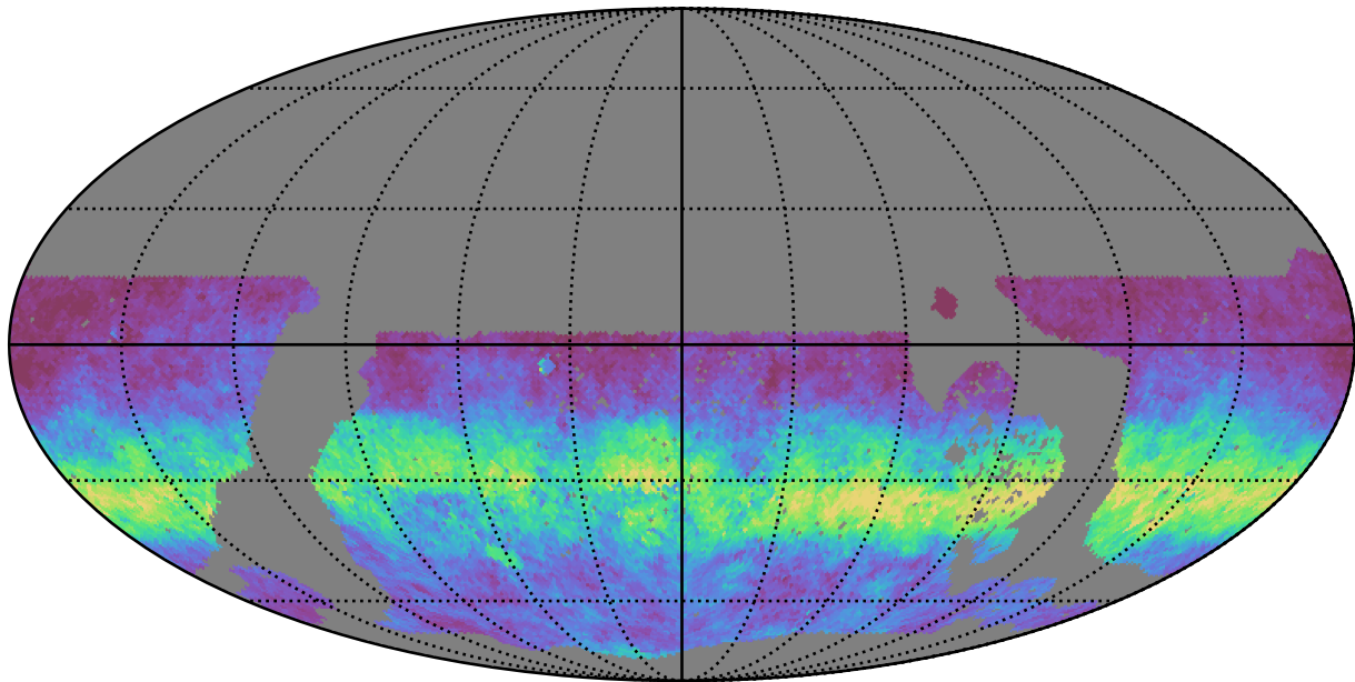
no_long_daily_v3.4_10yrs WFD g band: AngleRms rotSkyPos
