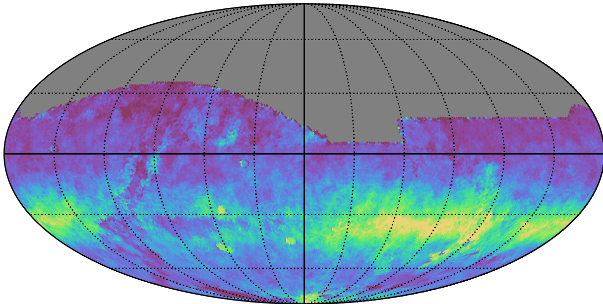
no_long_daily_v3.4_10yrs All sky z band: AngleRms rotSkyPos
