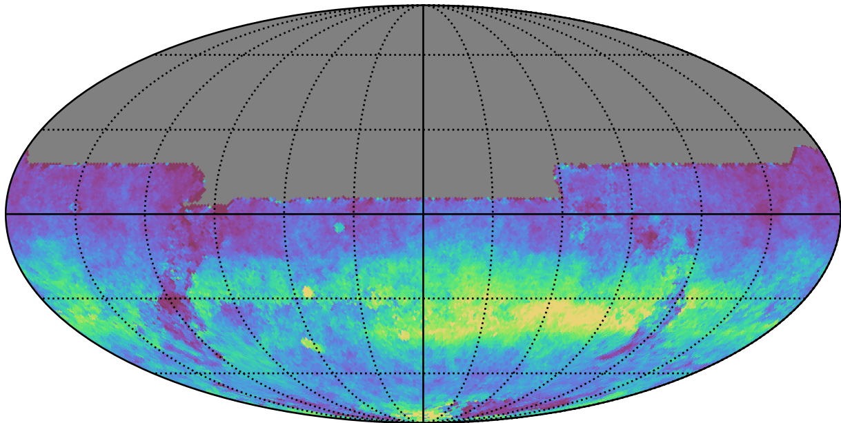
no_long_daily_v3.4_10yrs All sky y band: AngleRms rotSkyPos
