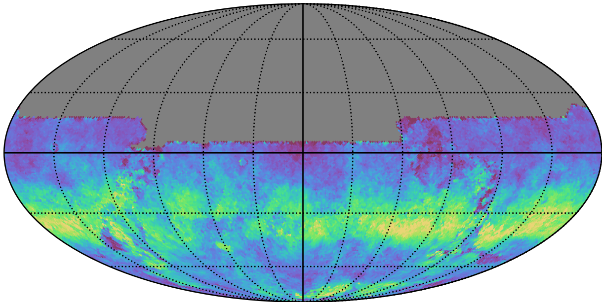
no_long_daily_v3.4_10yrs All sky u band: AngleRms rotSkyPos
