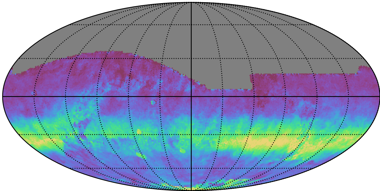
no_long_daily_v3.4_10yrs All sky r band: AngleRms rotSkyPos
