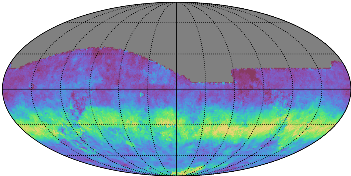
no_long_daily_v3.4_10yrs All sky g band: AngleRms rotSkyPos
