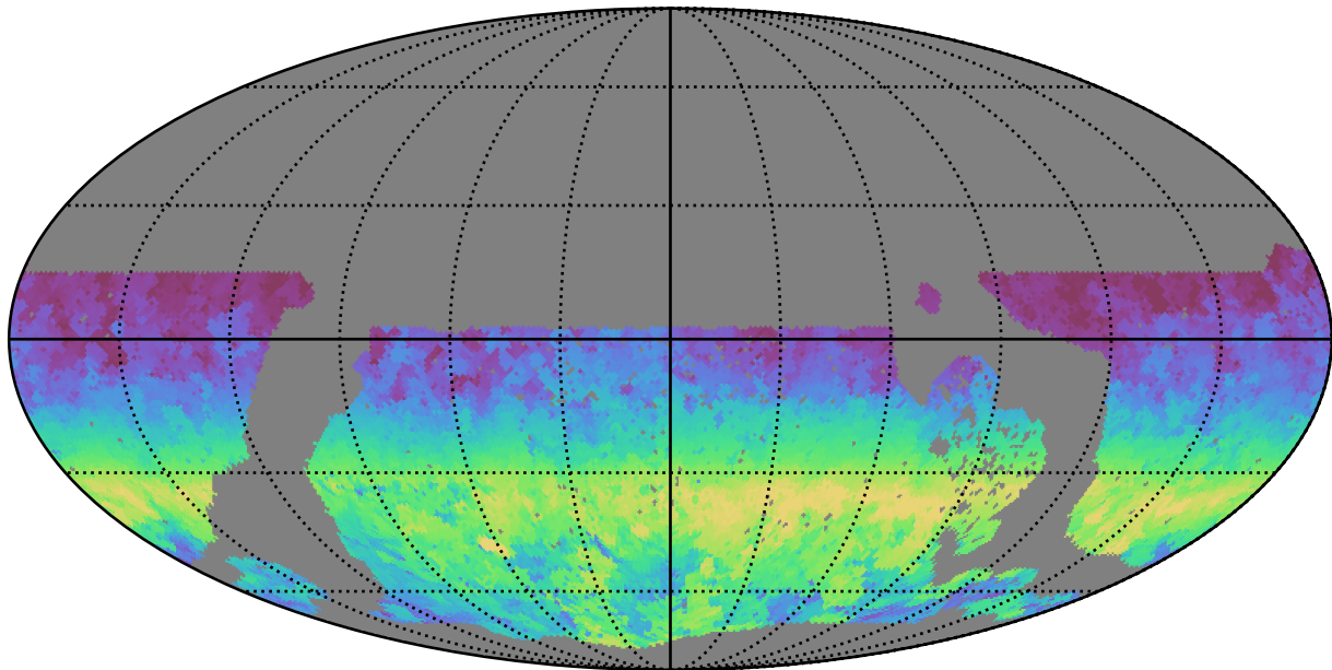
no_long_daily_v3.4_10yrs WFD z band: AngleRange rotSkyPos
