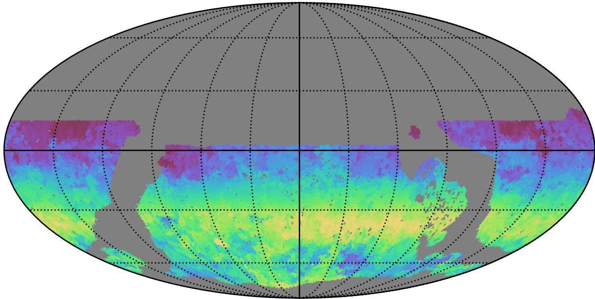
no_long_daily_v3.4_10yrs WFD y band: AngleRange rotSkyPos
