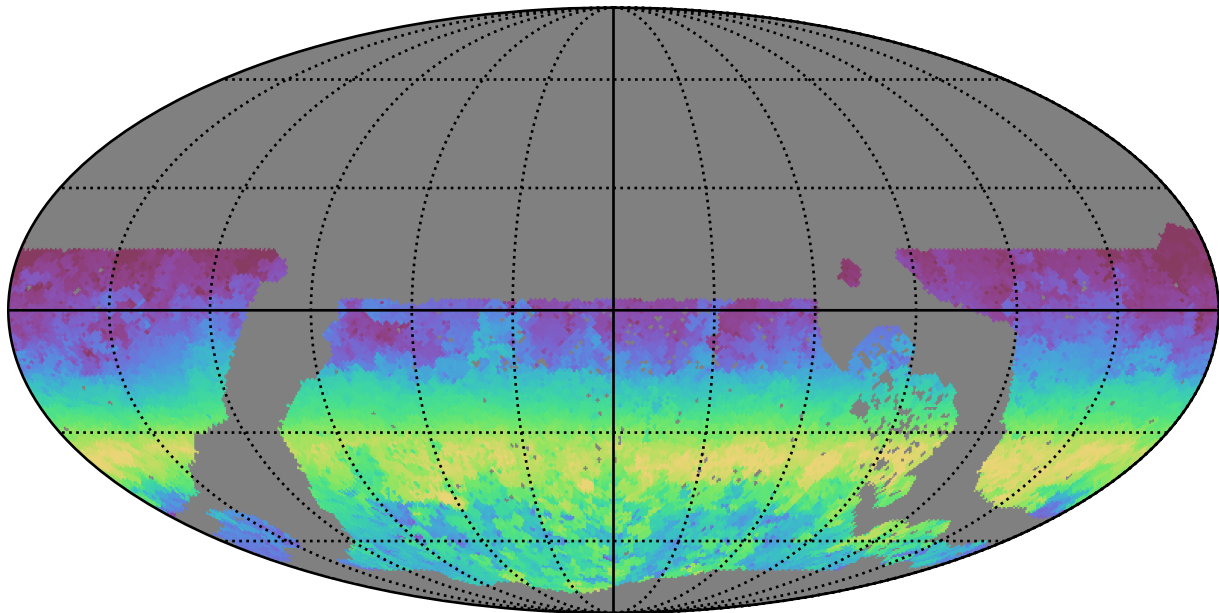
no_long_daily_v3.4_10yrs WFD r band: AngleRange rotSkyPos
