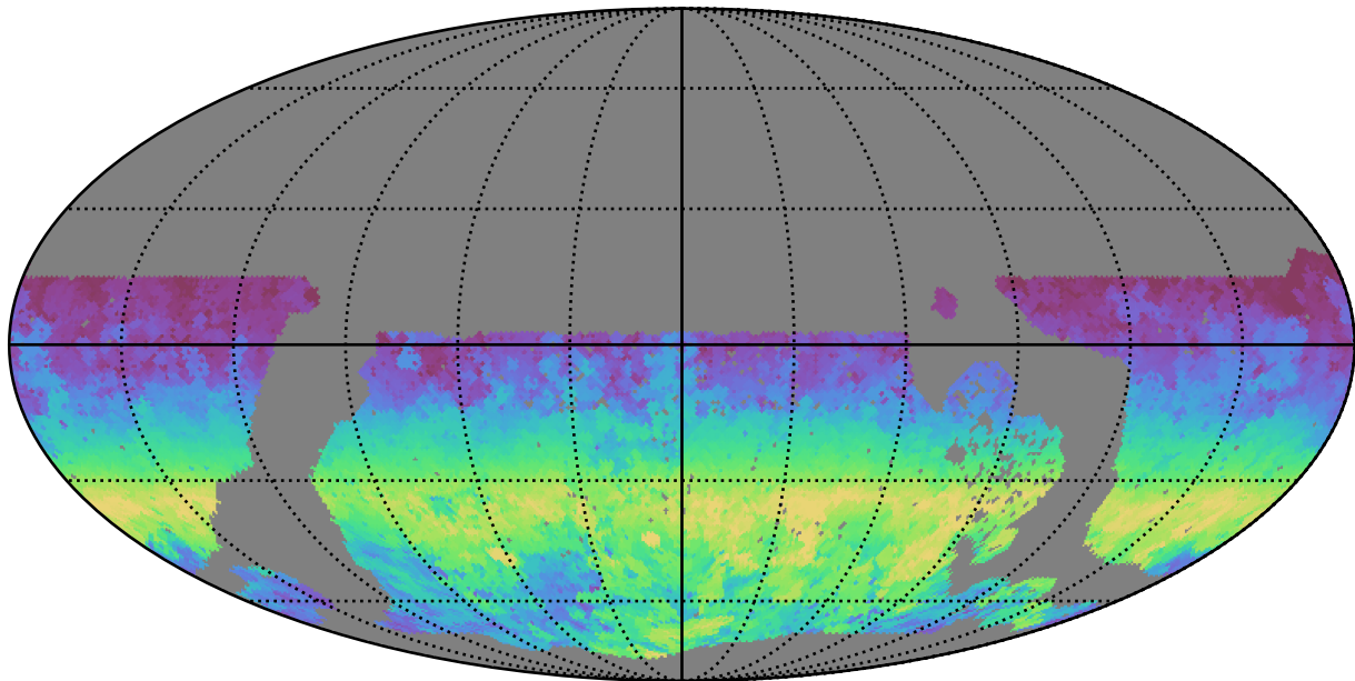
no_long_daily_v3.4_10yrs WFD i band: AngleRange rotSkyPos
