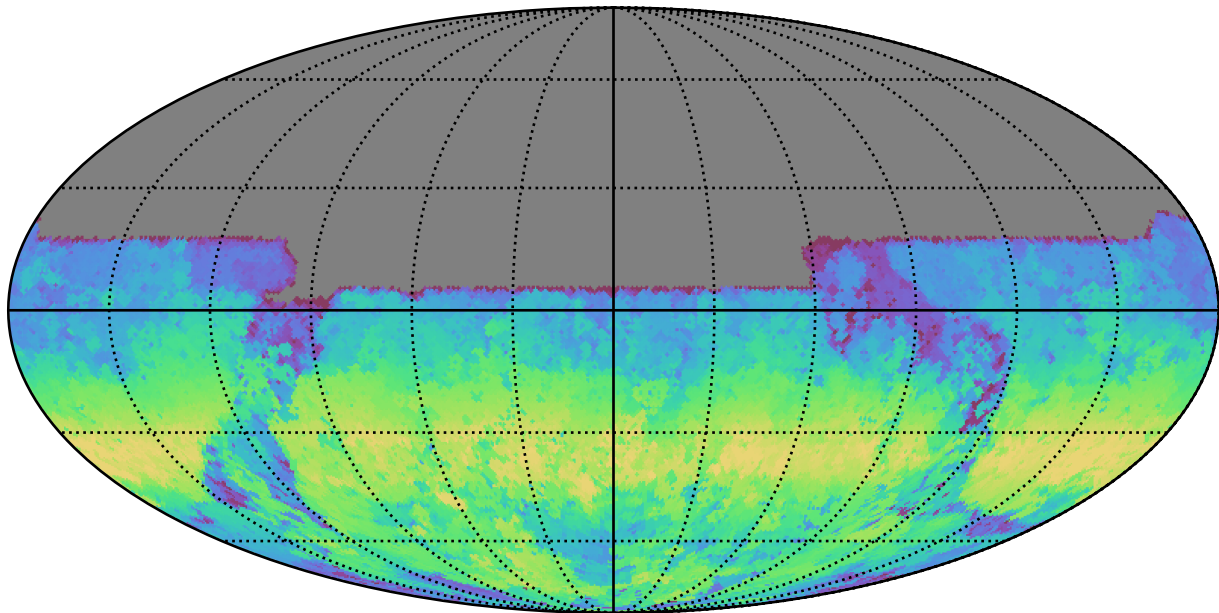
no_long_daily_v3.4_10yrs All sky u band: AngleRange rotSkyPos
