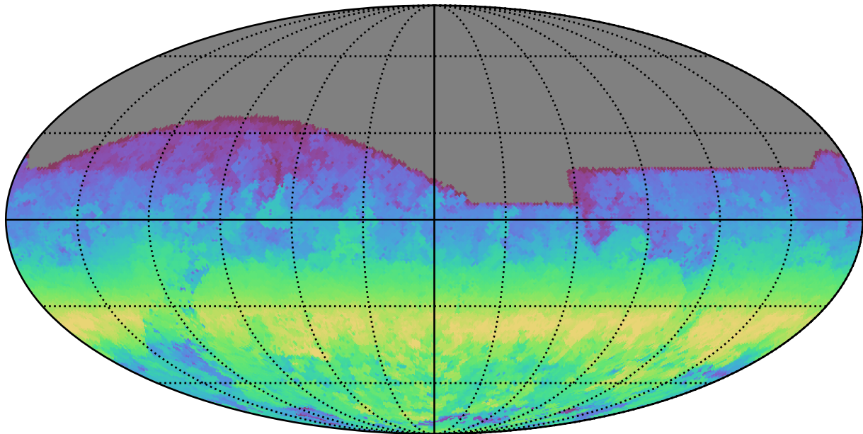
no_long_daily_v3.4_10yrs All sky r band: AngleRange rotSkyPos
