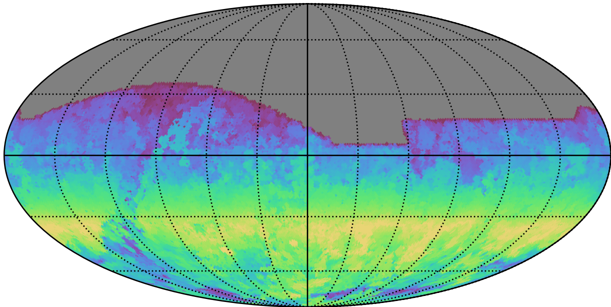
no_long_daily_v3.4_10yrs All sky i band: AngleRange rotSkyPos
