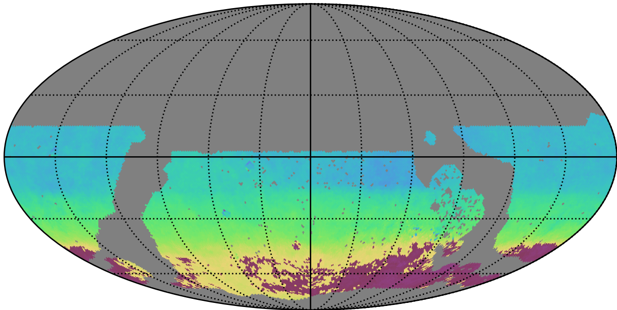
no_long_daily_v3.4_10yrs WFD z band: AngleMean rotSkyPos
