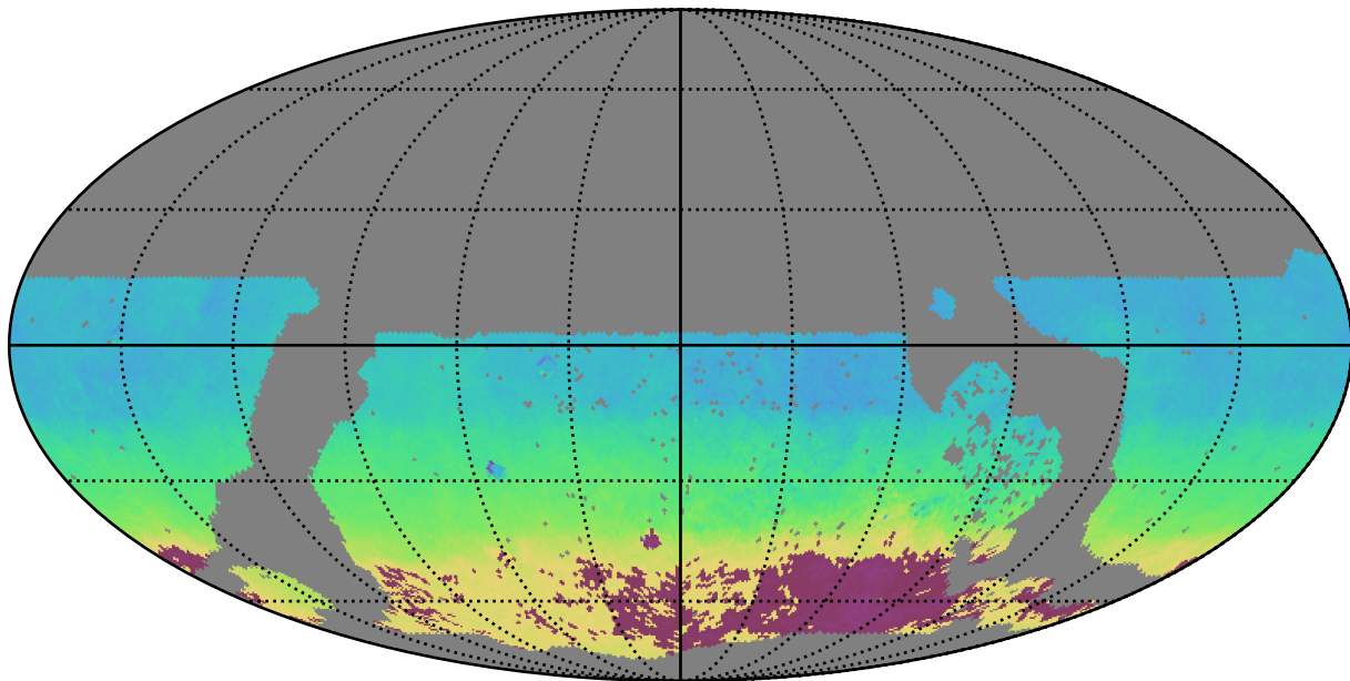
no_long_daily_v3.4_10yrs WFD y band: AngleMean rotSkyPos
