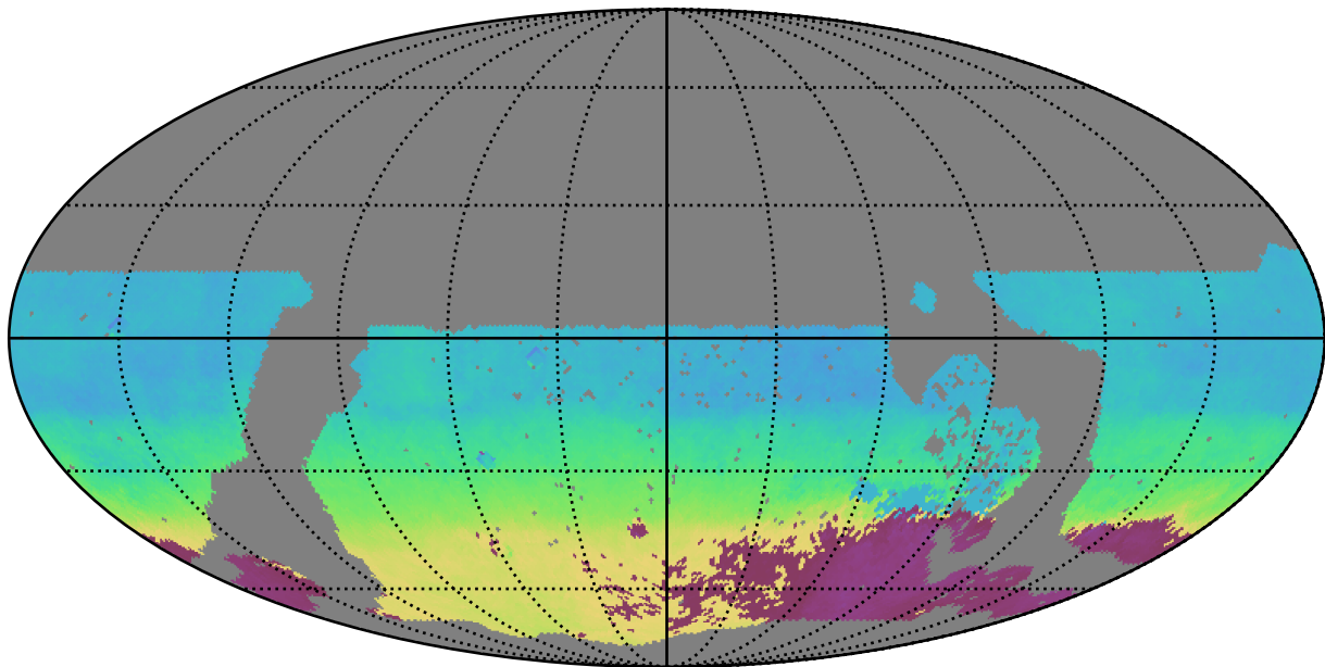
no_long_daily_v3.4_10yrs WFD r band: AngleMean rotSkyPos
