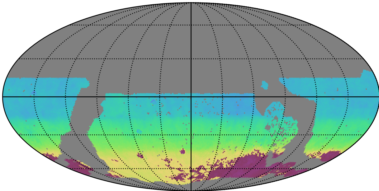
no_long_daily_v3.4_10yrs WFD i band: AngleMean rotSkyPos
