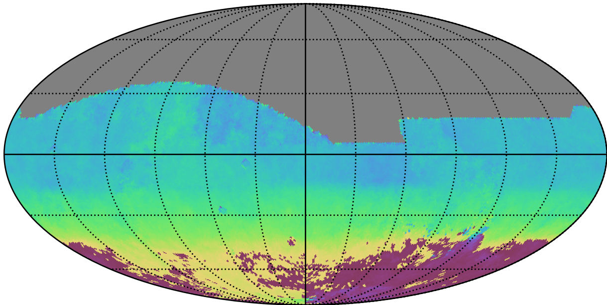
no_long_daily_v3.4_10yrs All sky z band: AngleMean rotSkyPos
