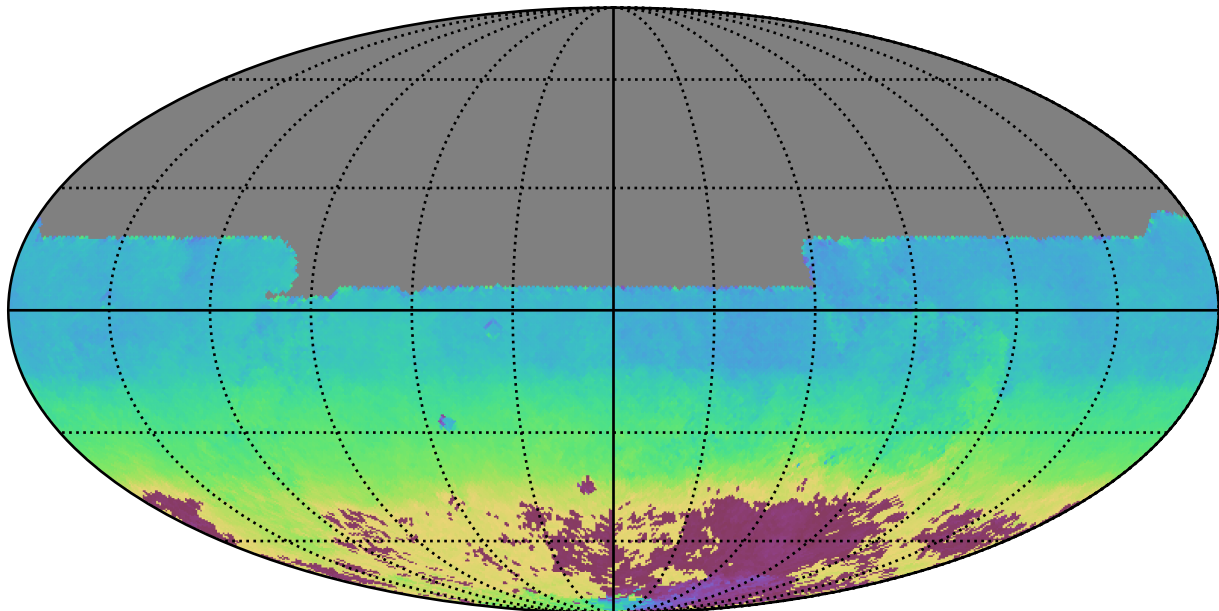
no_long_daily_v3.4_10yrs All sky y band: AngleMean rotSkyPos
