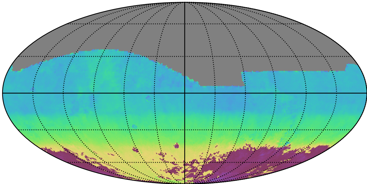
no_long_daily_v3.4_10yrs All sky i band: AngleMean rotSkyPos
