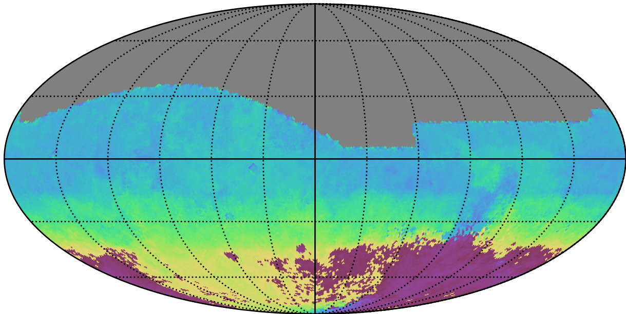
no_long_daily_v3.4_10yrs All sky g band: AngleMean rotSkyPos
