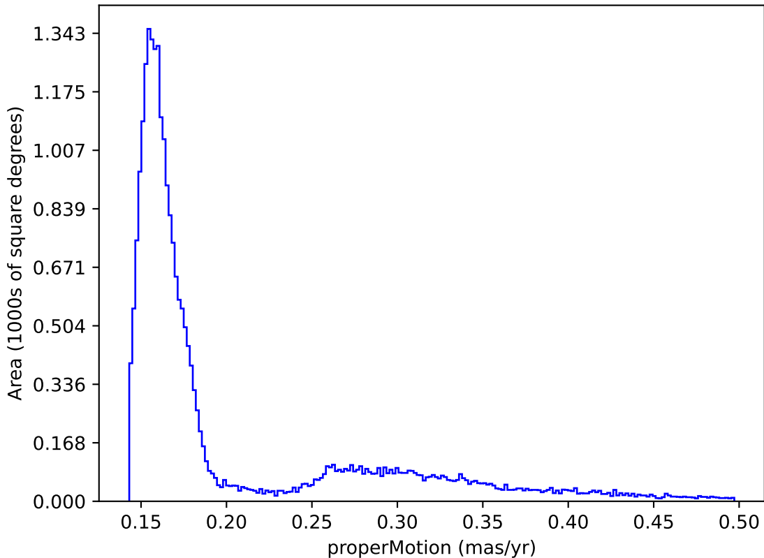
no_long_daily_v3.4_10yrs : properMotion
