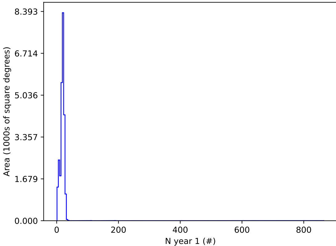
no_long_daily_v3.4_10yrs y and night &lt; 365: N year 1
