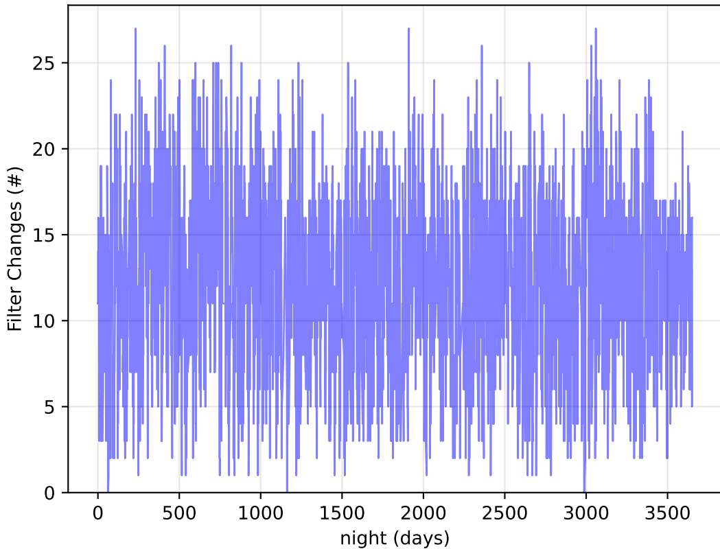
no_long_daily_v3.4_10yrs : Filter Changes
