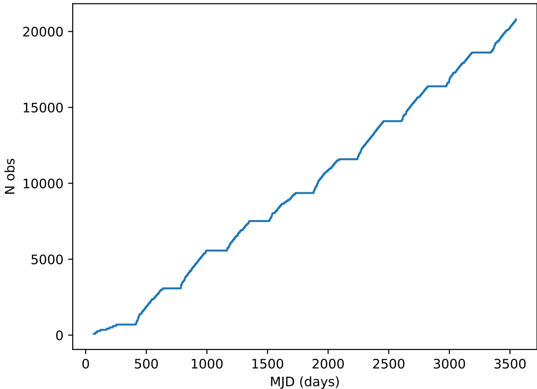
no_long_daily_v3.4_10yrs note like DD:ELAISS1%: Cumulative
