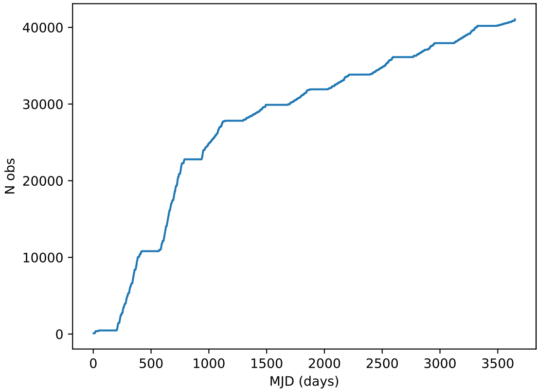
no_long_daily_v3.4_10yrs note like DD:COSMOS%: Cumulative
