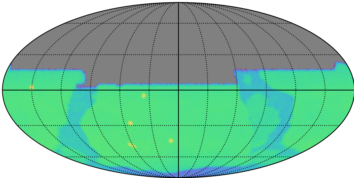
no_long_daily_v3.4_10yrs y: CoaddM5
