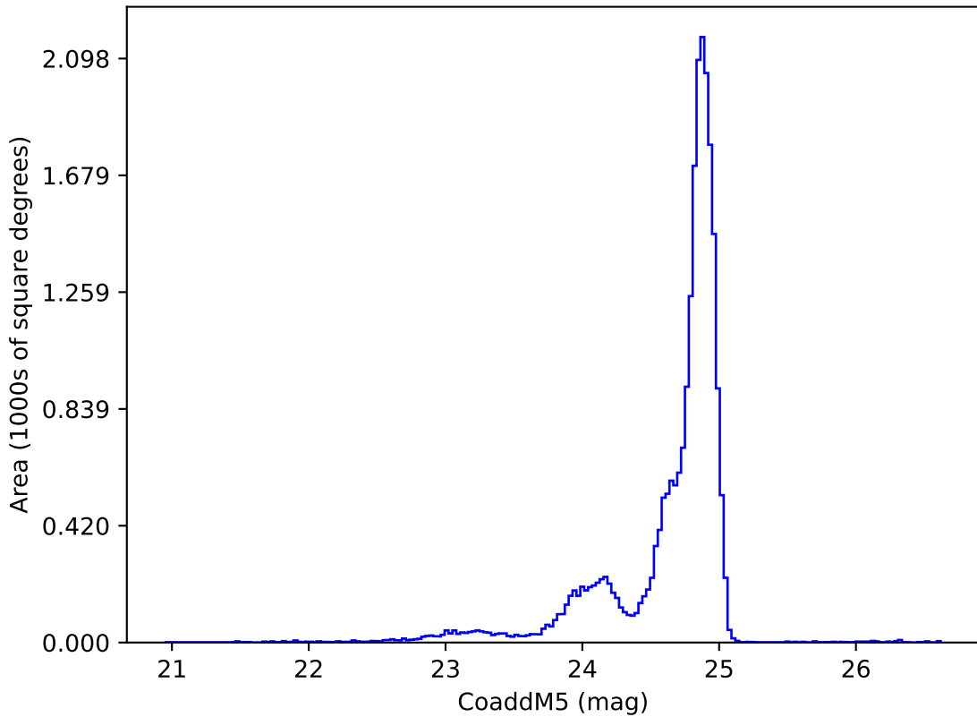
no_long_daily_v3.4_10yrs y: CoaddM5
