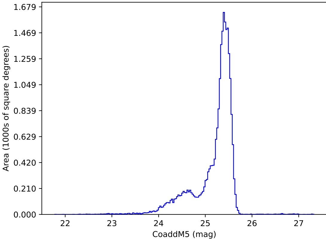
no_long_daily_v3.4_10yrs u: CoaddM5
