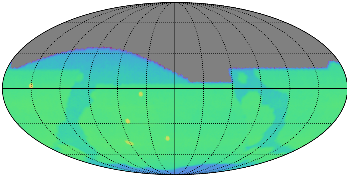
no_long_daily_v3.4_10yrs r: CoaddM5
