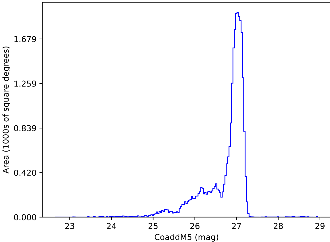
no_long_daily_v3.4_10yrs r: CoaddM5
